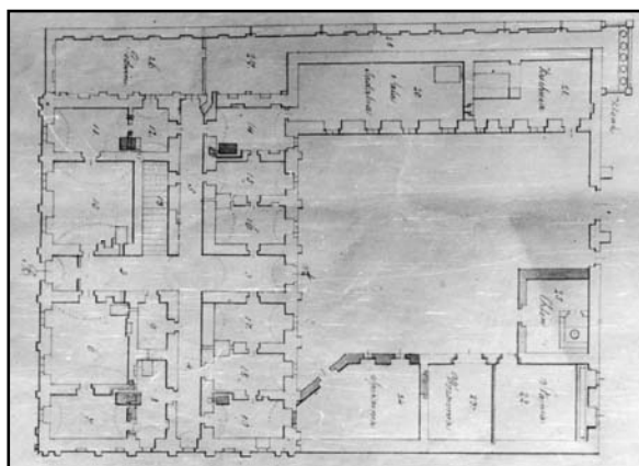
Foto 12. Plan parteru gmachu seminaryjnego
