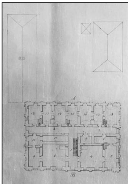
Foto 13. Plan piętra budynku seminaryjnego
