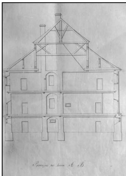
Foto 11. Przekrój pionowy budynku seminarium
